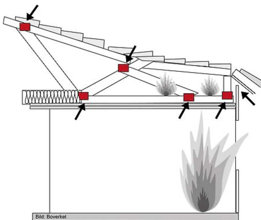
Exempel på svaga punkter i byggnadens brandskydd. (Boverket)
