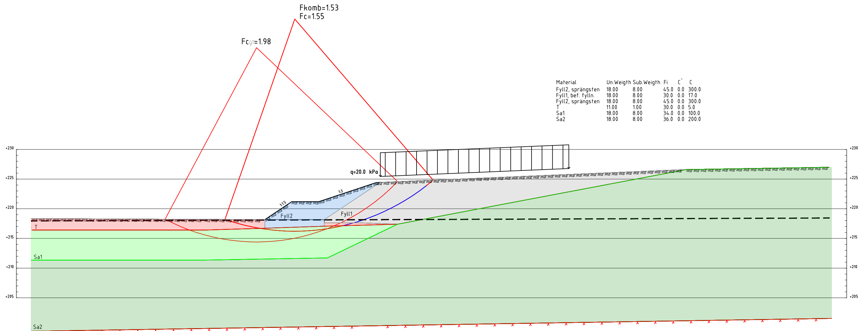
SEKTION A-A, SLUTLIG SLÄNT 1:200 (A1), 1:400 (A3)
