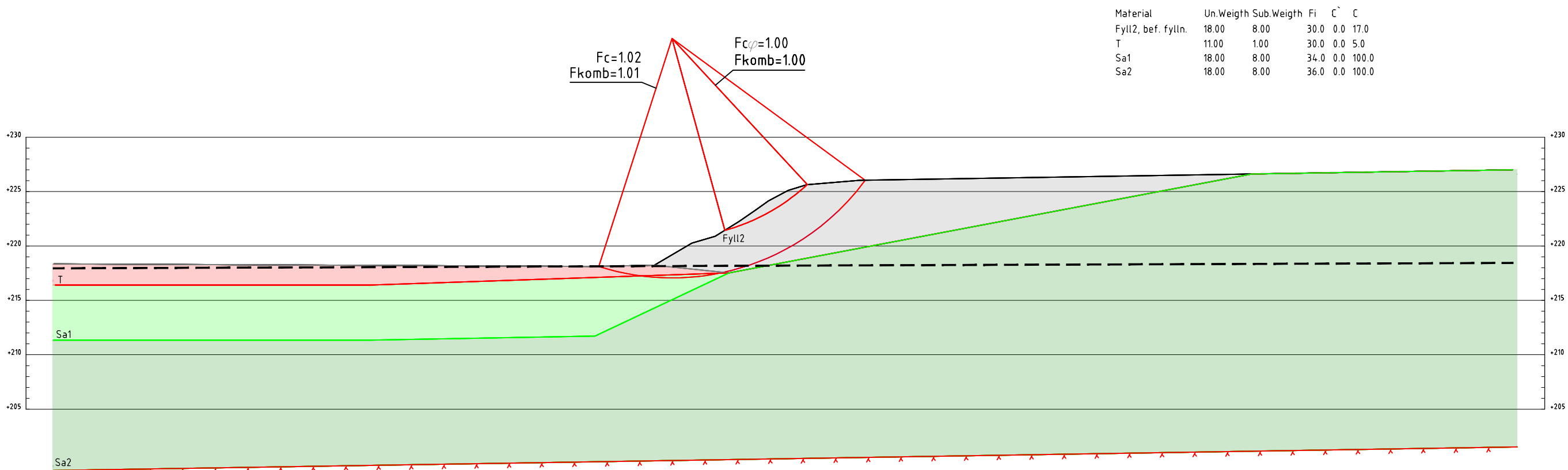
SEKTION A-A, BEF. SLÄNT 1:200 (-1), 1:400 (-3)
