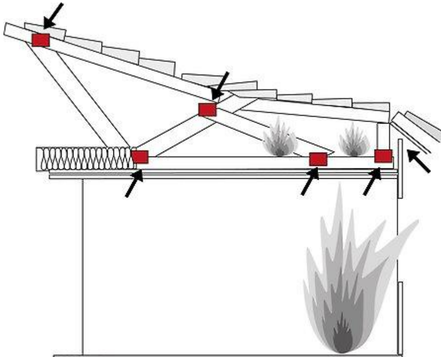
Exempel på svaga punkter i byggnadens brandskydd. (Boverket)
