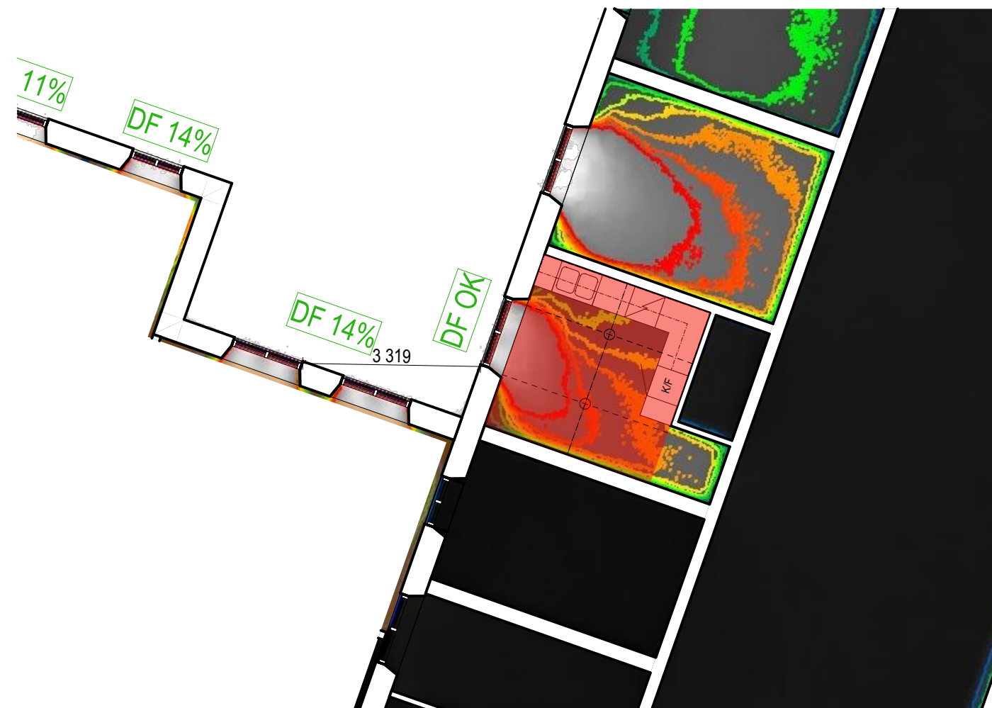
Plan 11 DAGSLJUS 1:100
