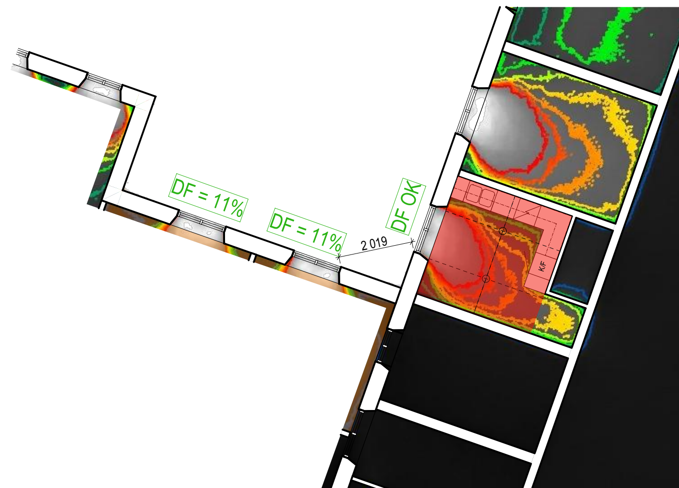
Plan 11 DAGSLJUS 1:100
