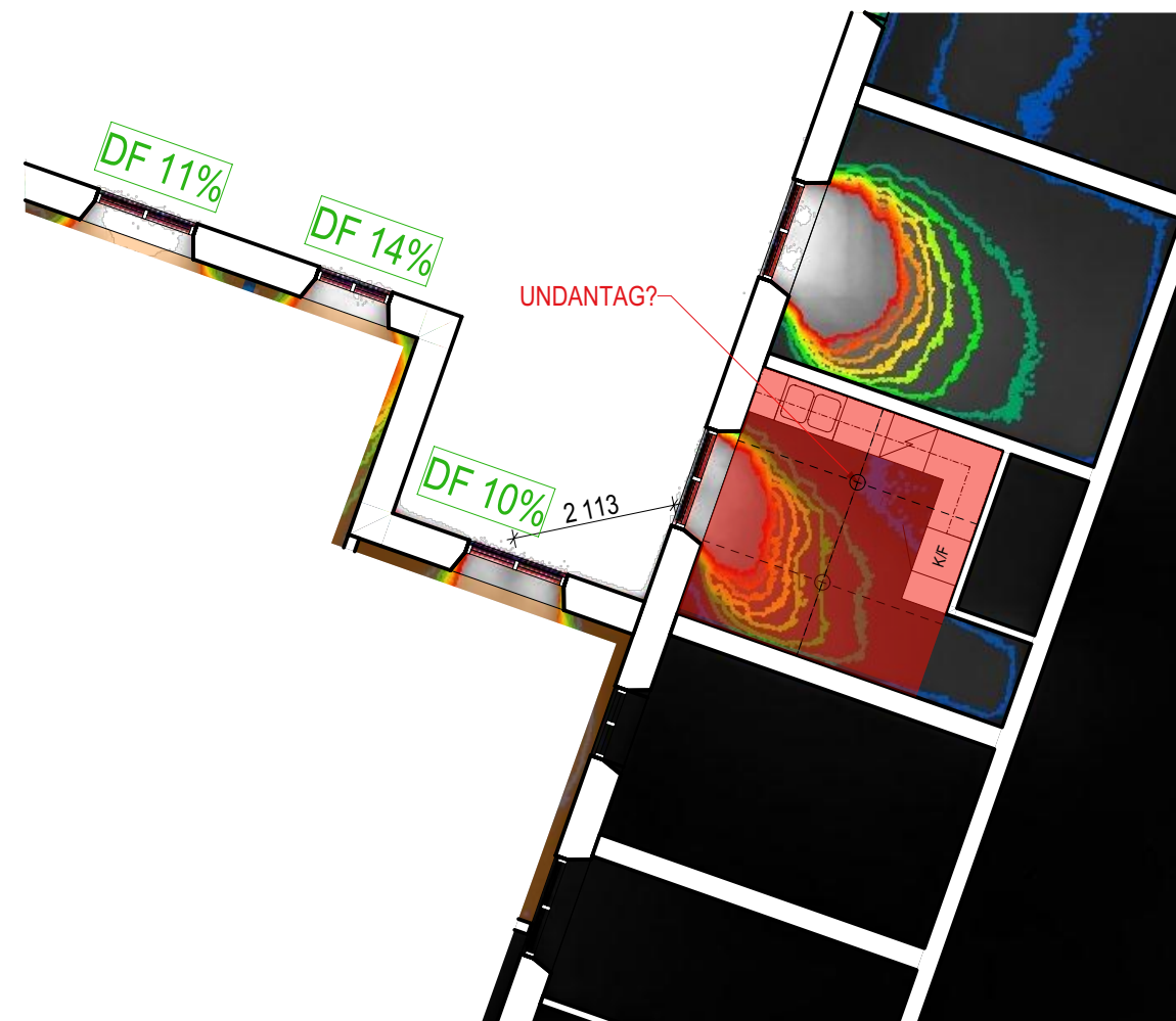
Plan 11 DAGSLJUS 1:100
