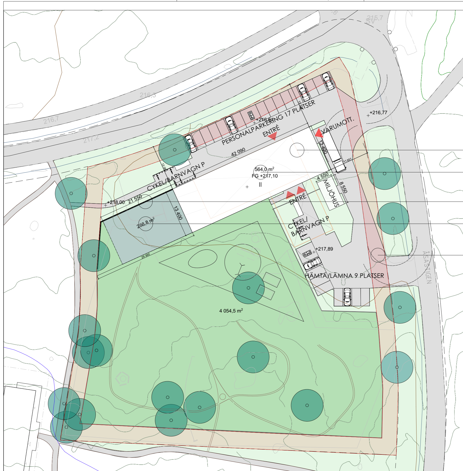
PLANSKISS 1:500
