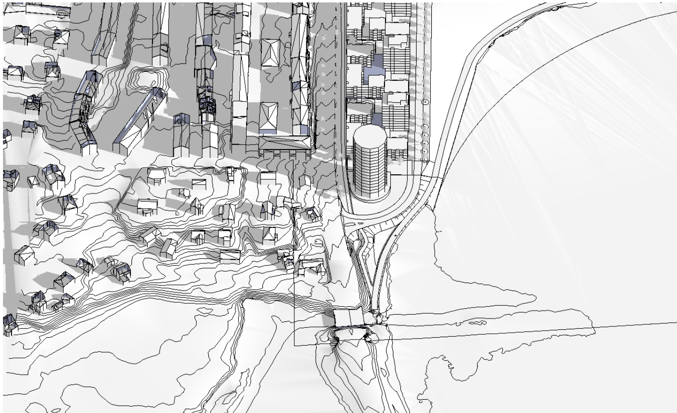
Vårdagjämning kl 09:00
