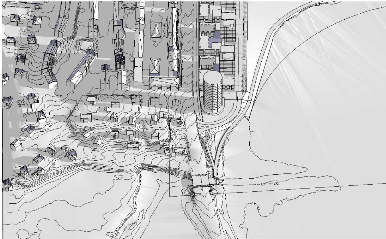
Vårdagjämning kl 08:00
