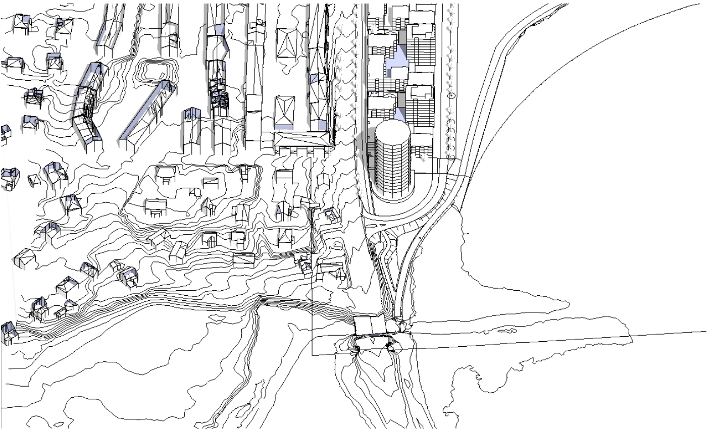
Midsommar kl 12:00
