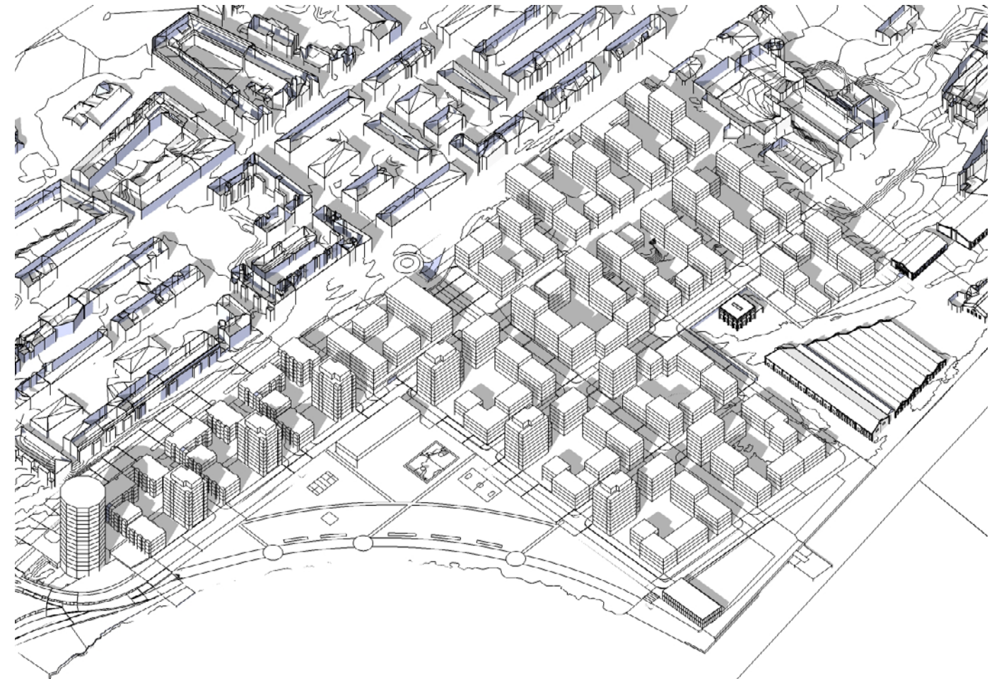
Vårdagjämning 12:00
