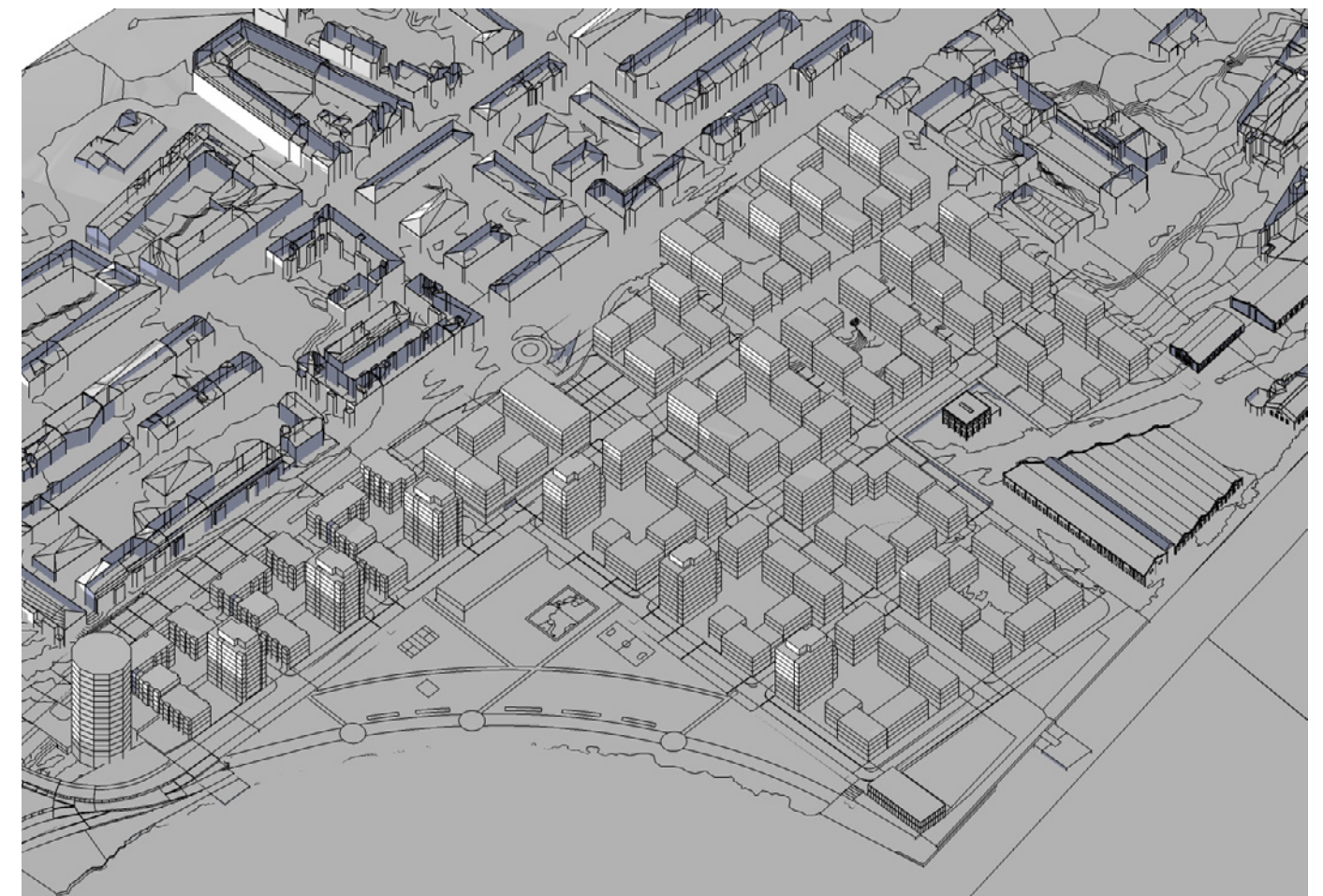
Vårdagjämning 18:00
