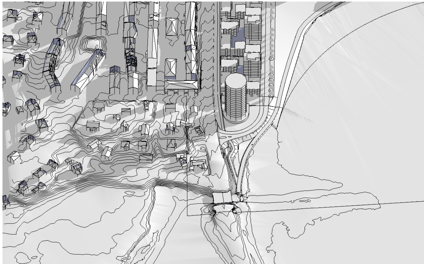
Midsommar kl 06:00
