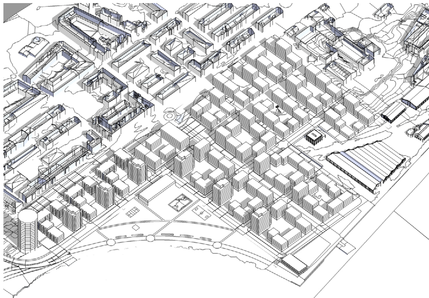
Midsommar 9:00
