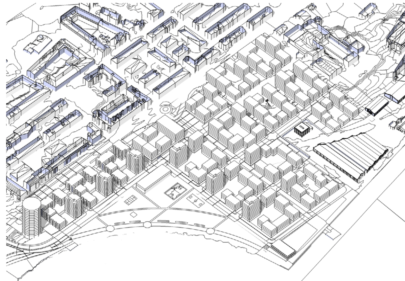
Midsommar 12:00
