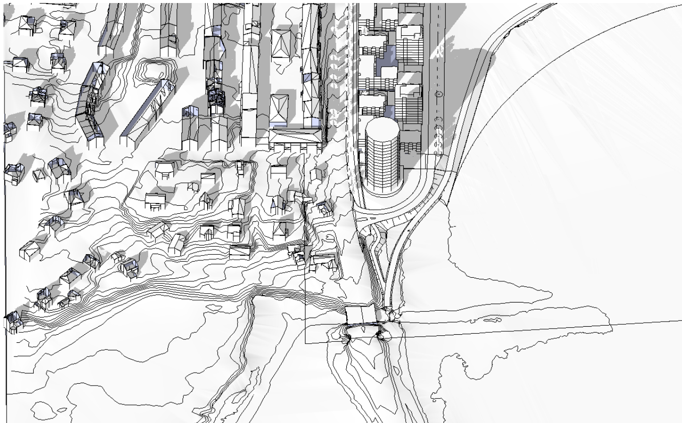
Vårdagjämning kl 15:00
