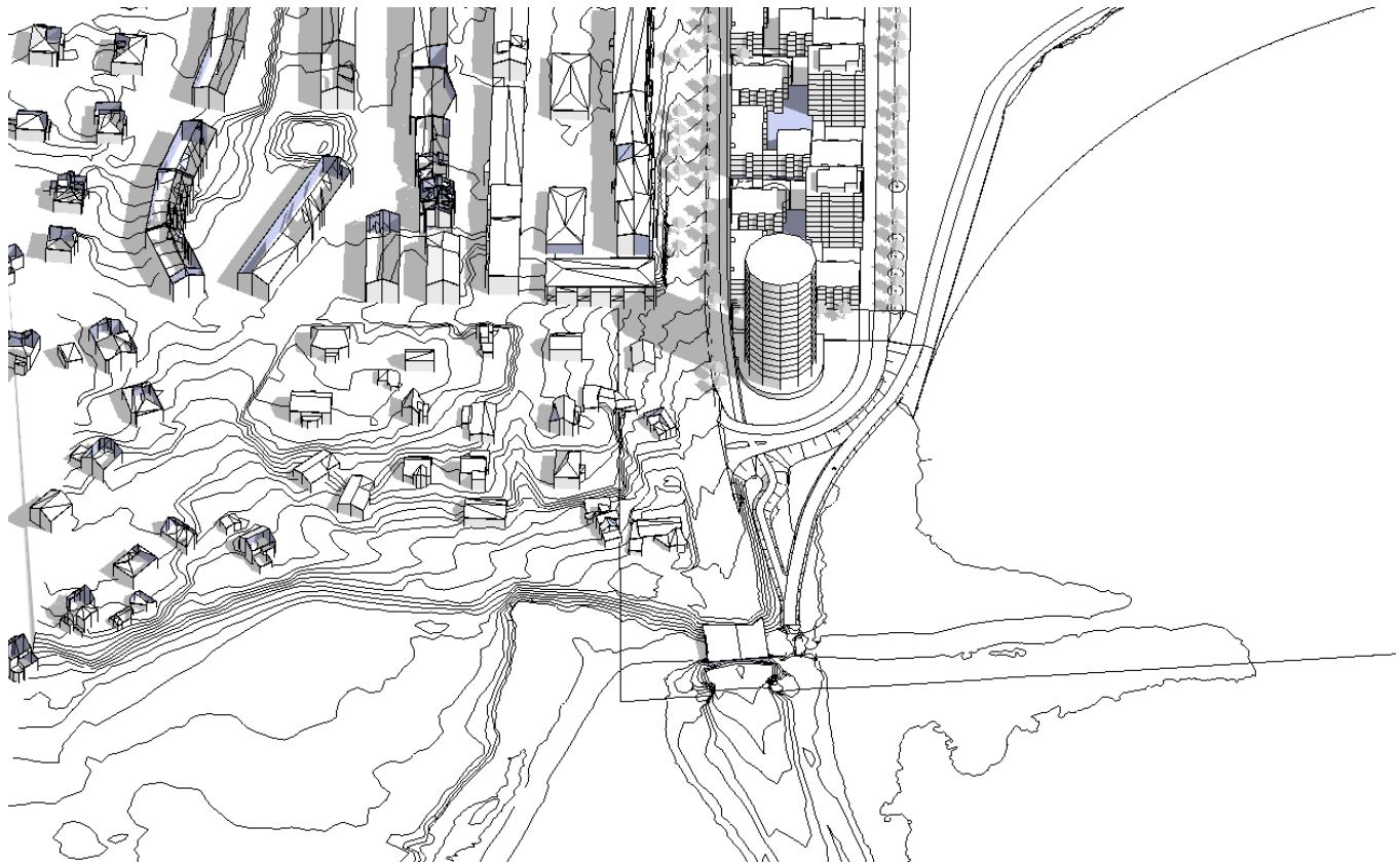
Midsommar kl 10:00
