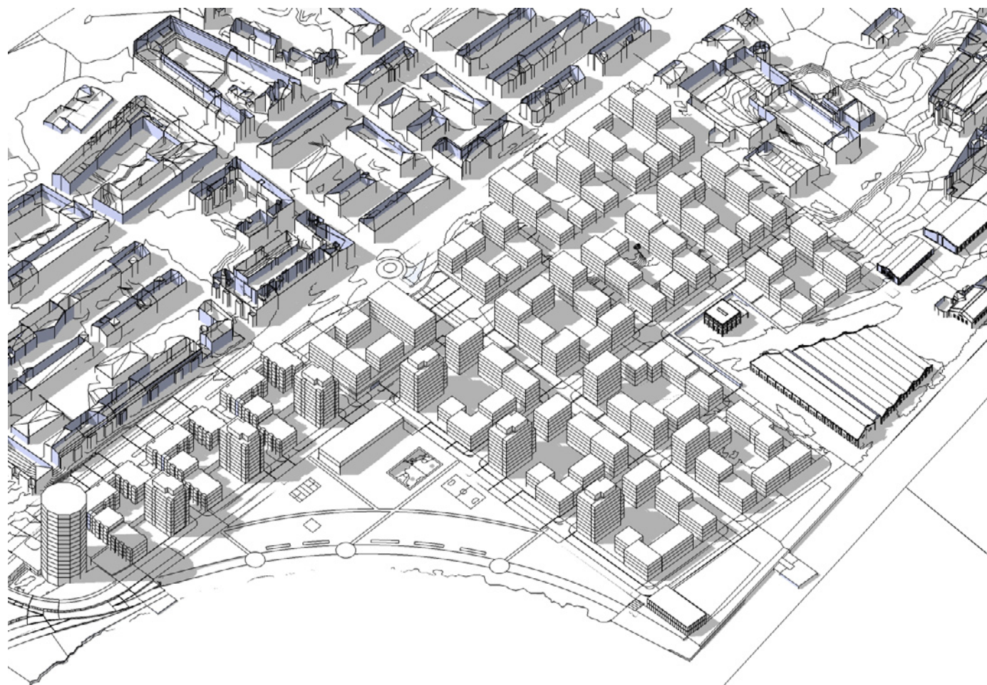
Midsommar 15:00
