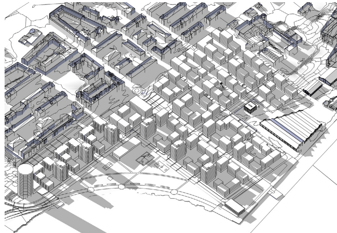
Midsommar 18:00
