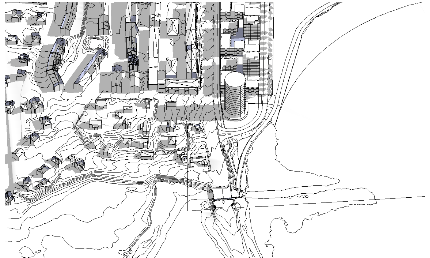
Midsommar kl 08:00
