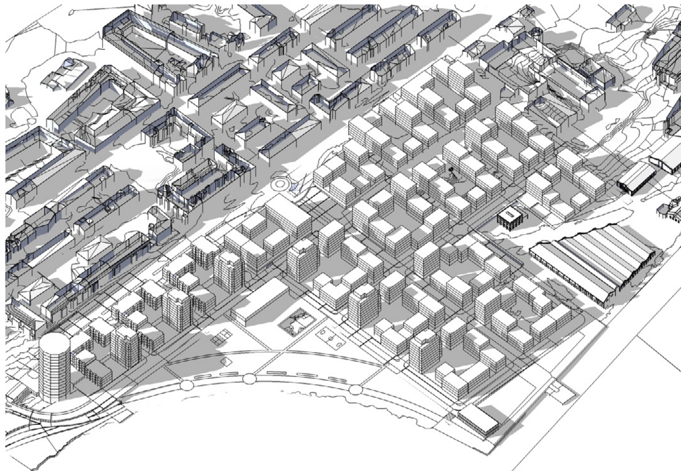
Vårdagjämning 15:00
