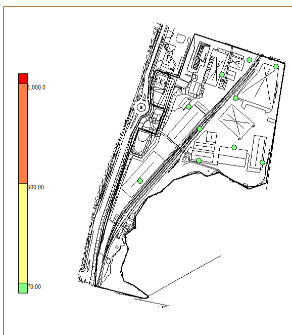
Figur 6 Översikt över provtagningspunkter för asfalt. Färgskalan anger uppmätt halt PAH16 (mg/kg TS) i dessa asfaltprover
