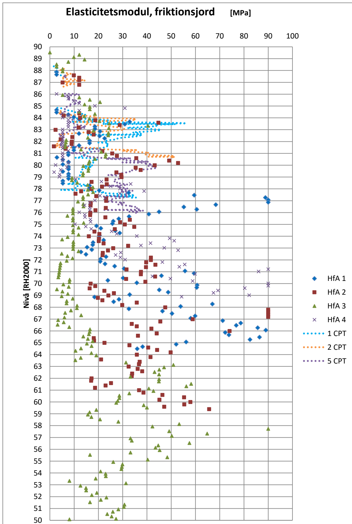
Figur 3 Utvärderad E-modul
