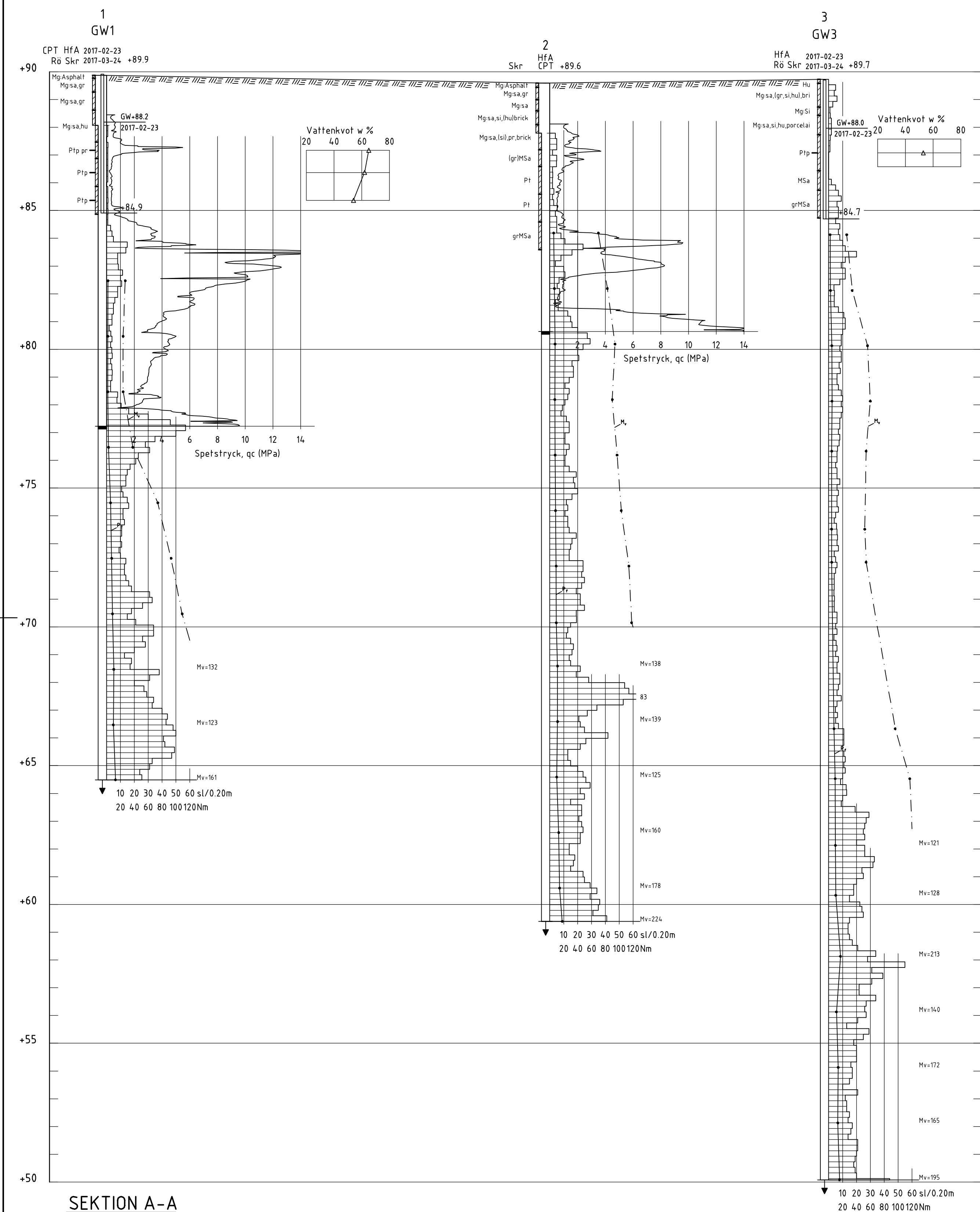
SEKTION A-A H 1: 100 L 1: 500
