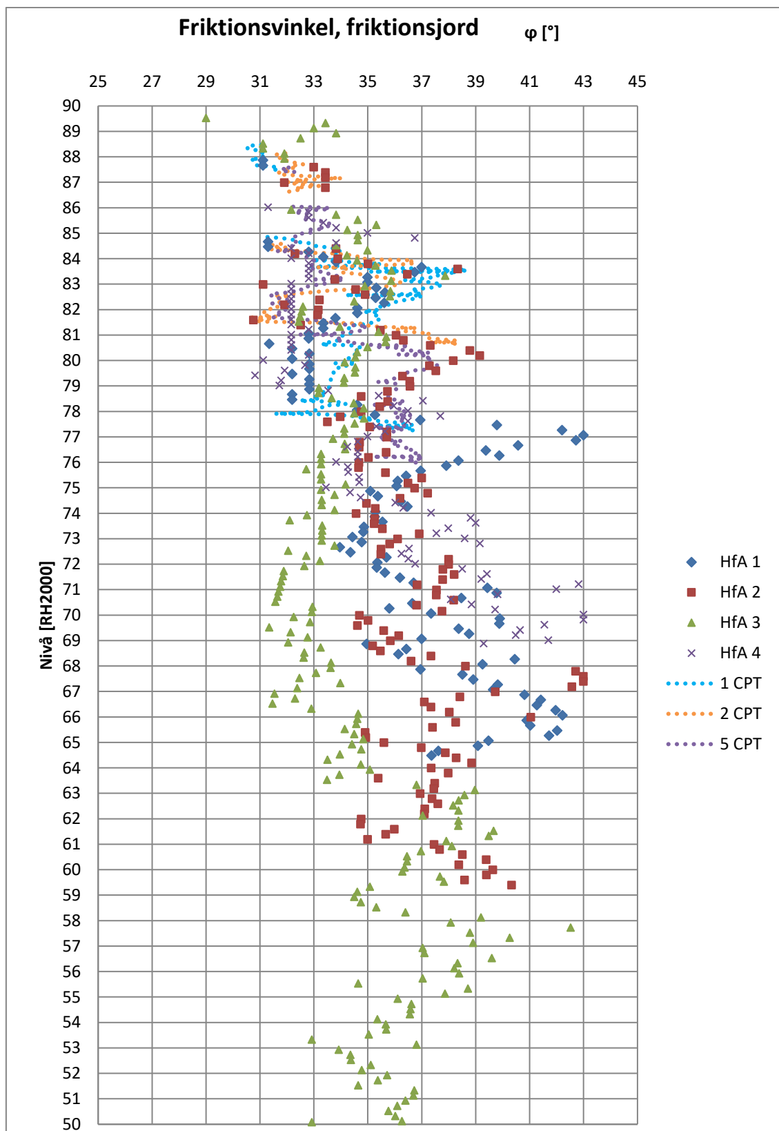
Figur 2 Utvärderad Friktionsvinkel
