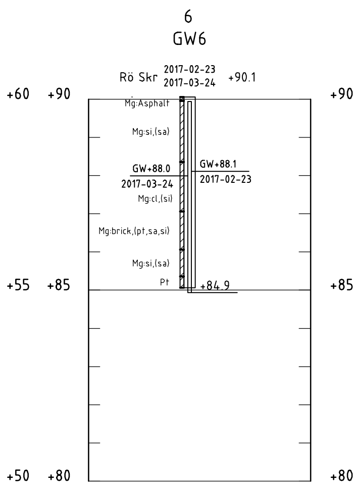
SEKTION C-C H 1: 100 L 1: 500
