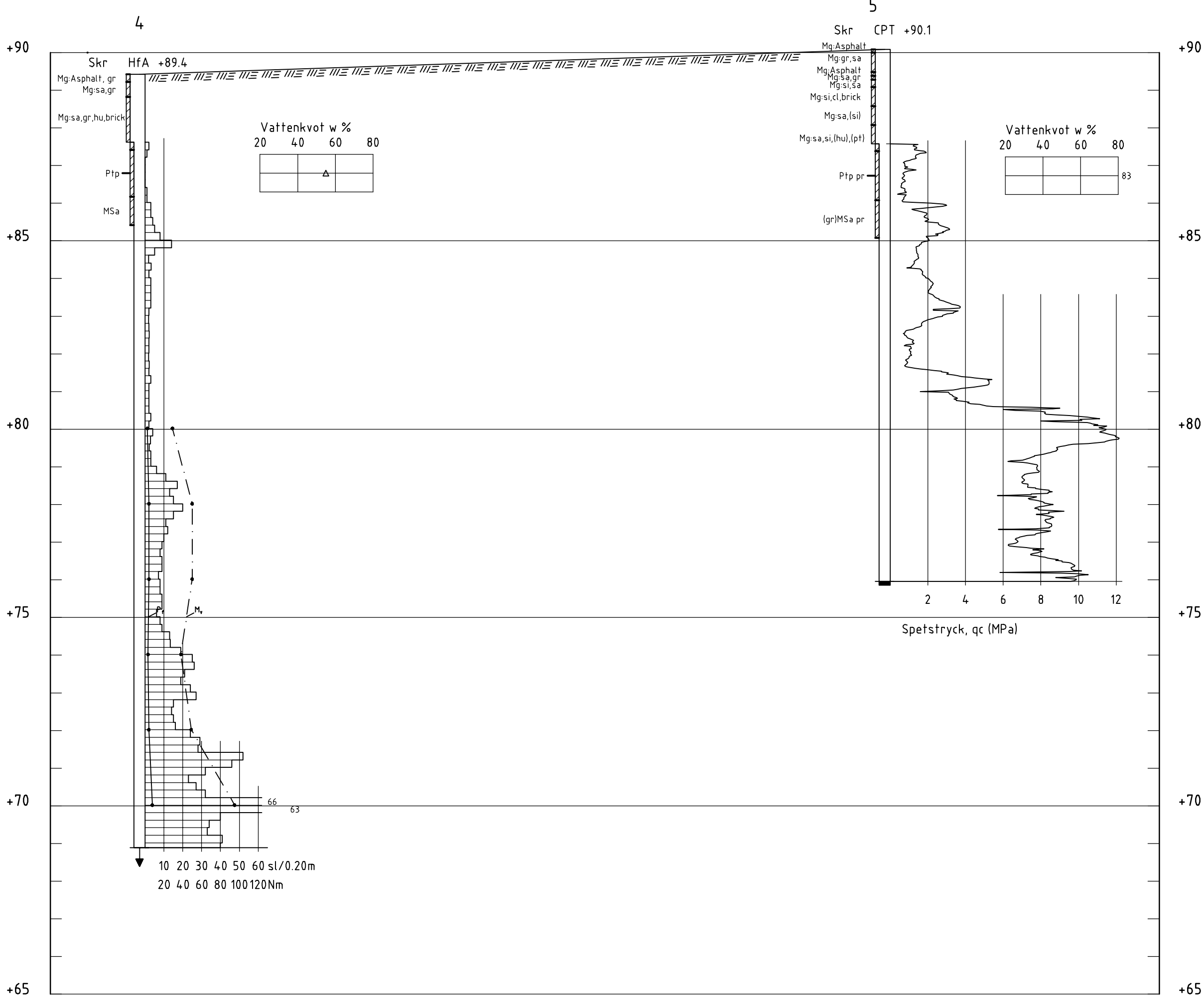
SEKTION B-B H 1: 100 L 1: 500
