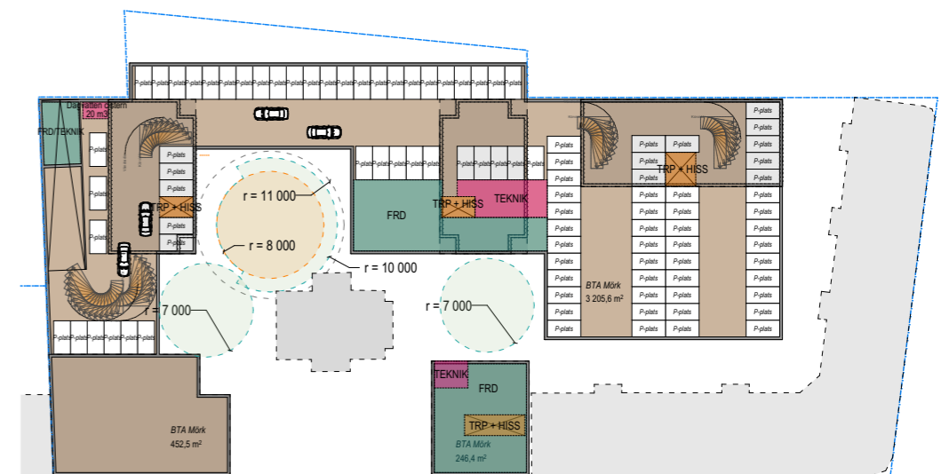
Plan 1 - Källarplan (Garage)
