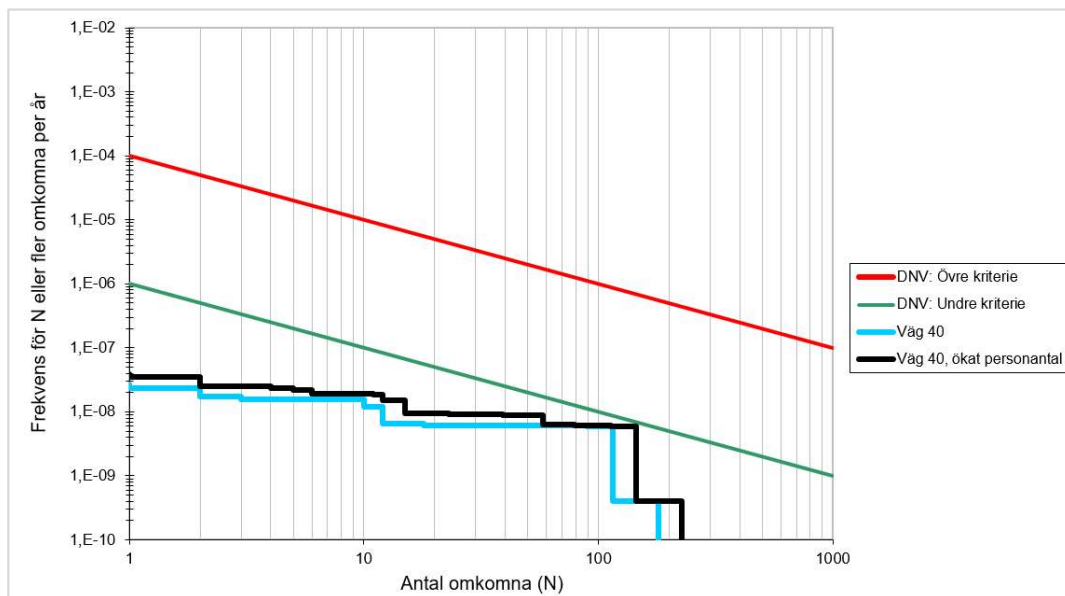
Figur 8. Förändring av samhällsrisknivå då personantalet höjs från 1900 till 2400 personer/km².
