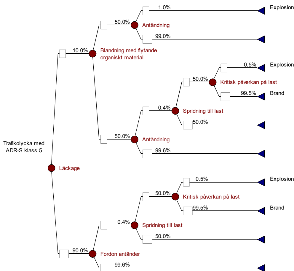
Figur 13. Händelseträd med sannolikheter för ADR-S klass 5.
