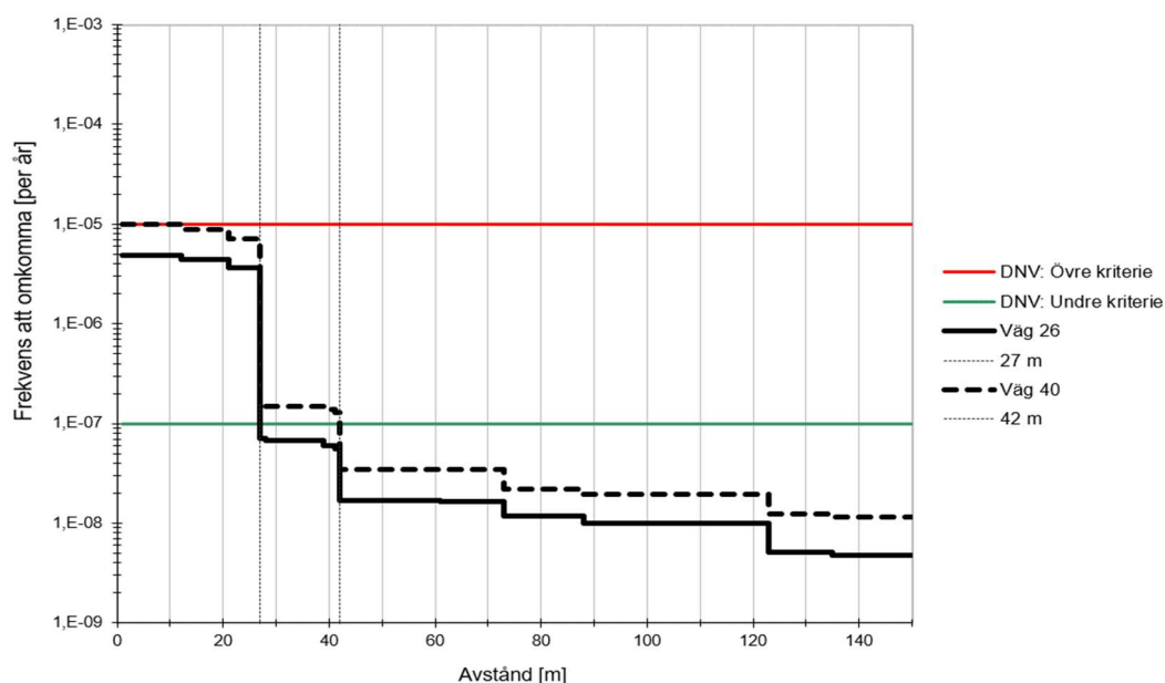
Figur 5. Individrisknivå med avseende på farligt gods-transporter på väg 26 respektive väg 40.
