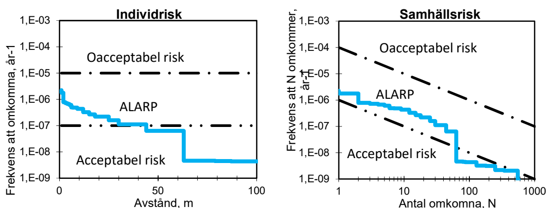
Figur 3. Föreslagna kriterier på individrisk samt samhällsrisk enligt DNV [8].
