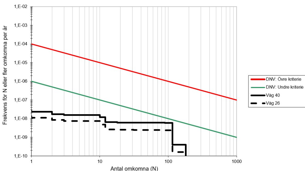
Figur 6. Samhällsrisk med avseende på väg 40 respektive väg 26.
