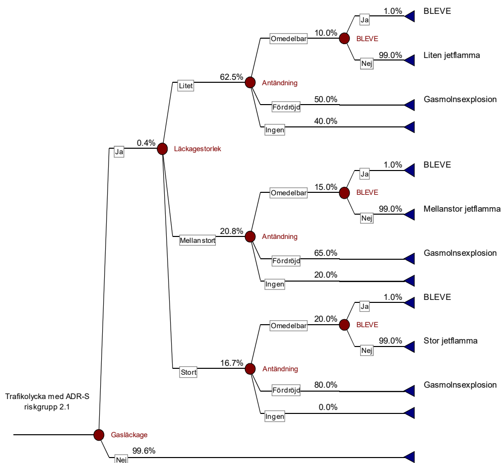
Figur 10. Händelseträd med sannolikheter för ADR-S klass 2.1.
