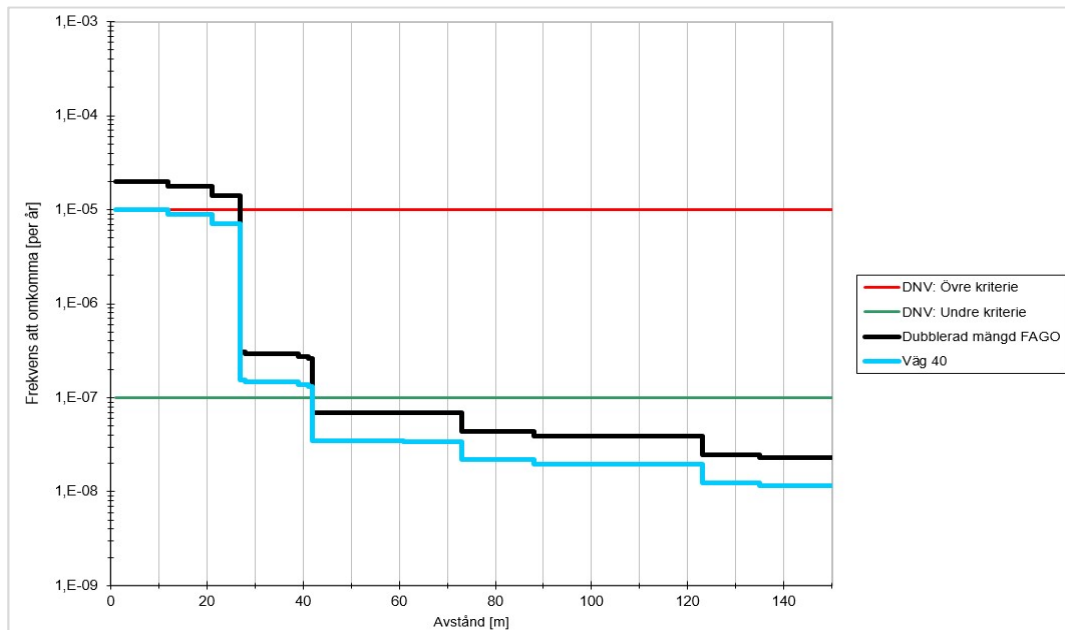
Figur 7. Förändring av individrisknivå då mängden farligt gods-transporter fördubblas.
