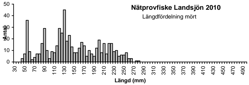
Figur 7. Längdfördelningsdiagram mört
