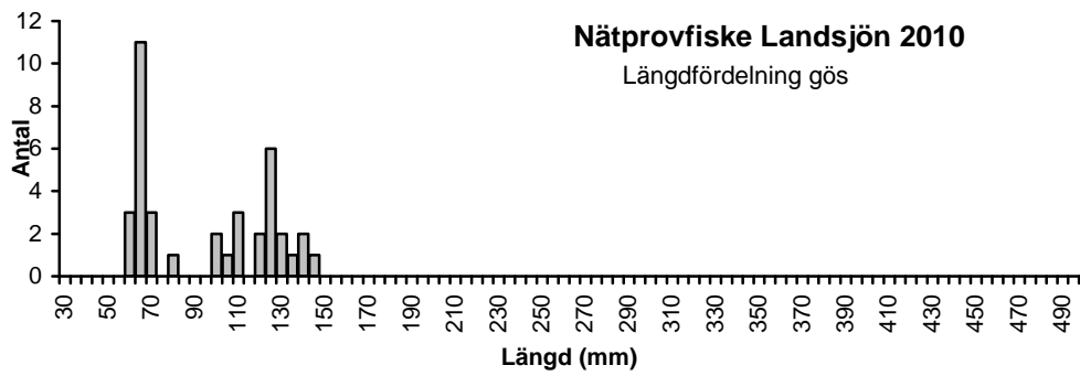
Figur 6. Längdfördelningsdiagram gös
