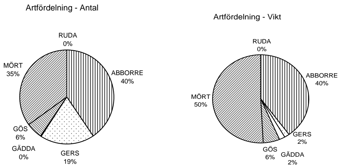
Figur 2. Artfördelningsdiagram
