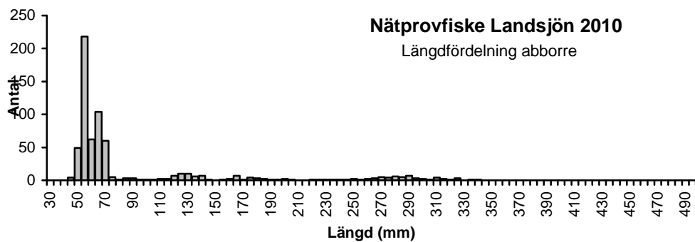
Figur 3. Längdfördelningsdiagram abborre
