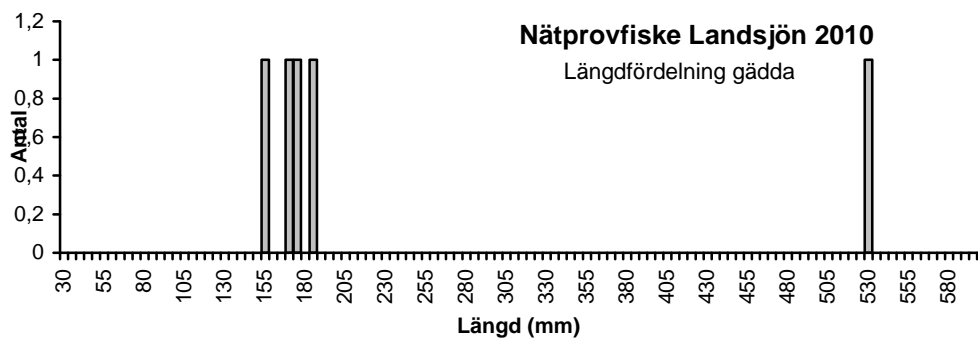
Figur 5. Längdfördelningsdiagram gädda
