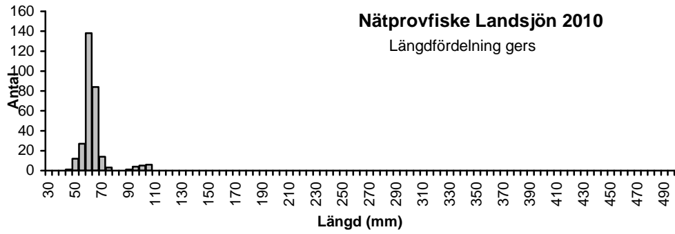
Figur 4. Längdfördelningsdiagram gers
