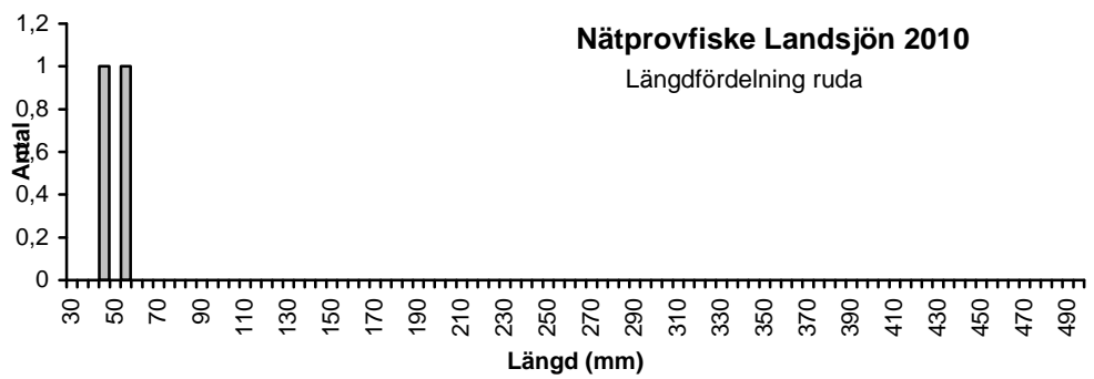
Figur 8. Längdfördelningsdiagram ruda
